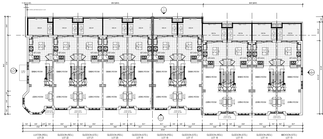
FIRST FLOOR SCALE: 1/8" = 1'-0"
