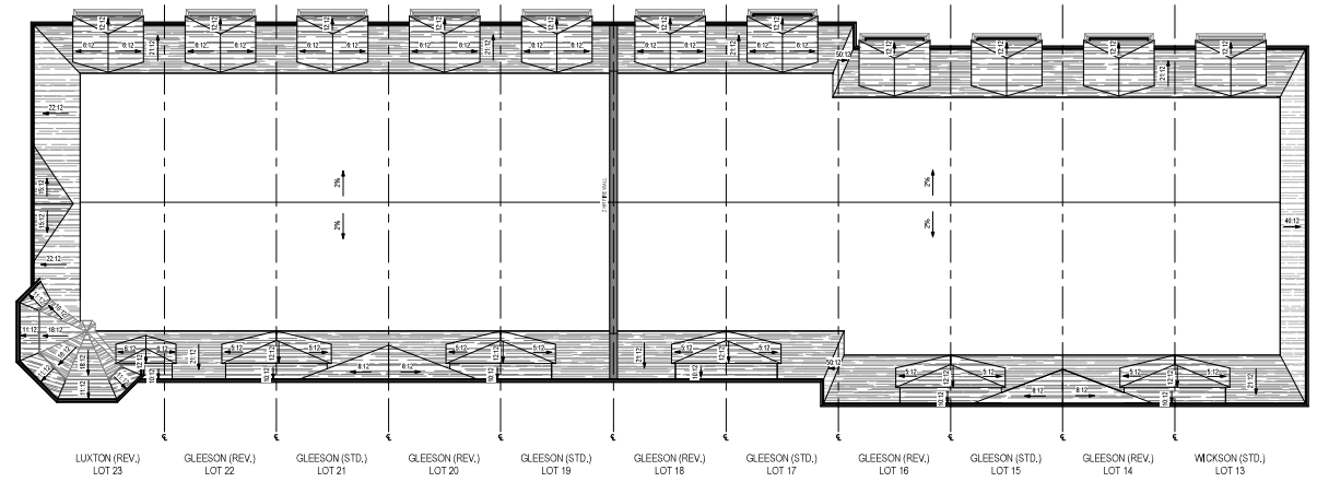
1 A20 ROOF PLAN SCALE: 1/8" = 1'-0"
