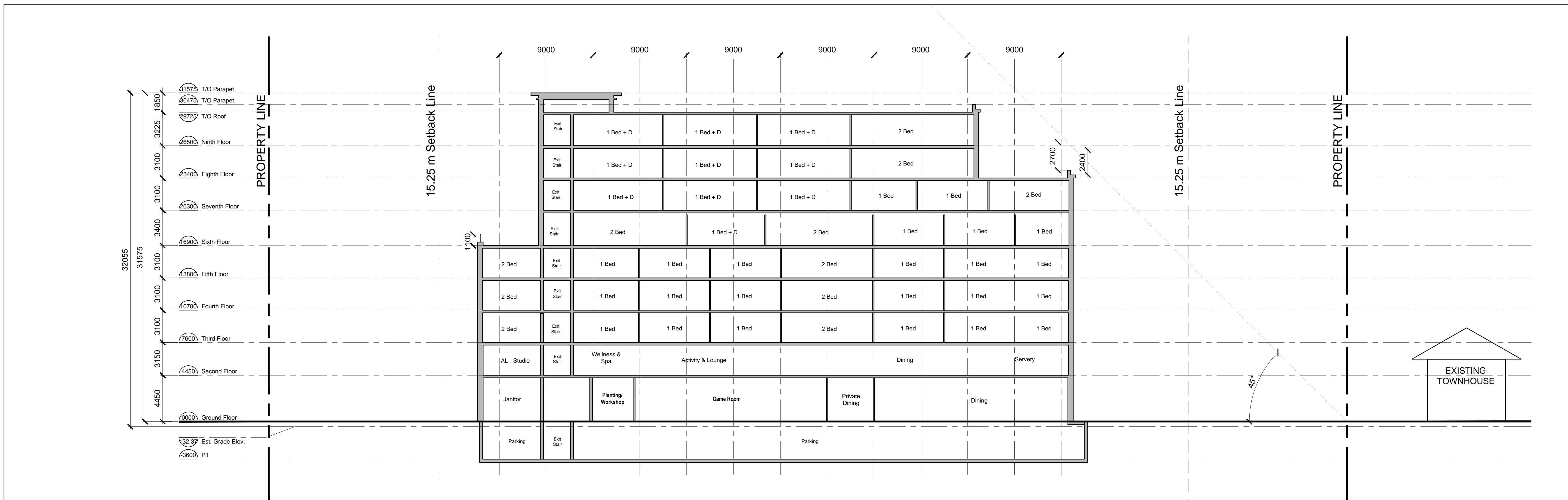
2 Section B-B A301
