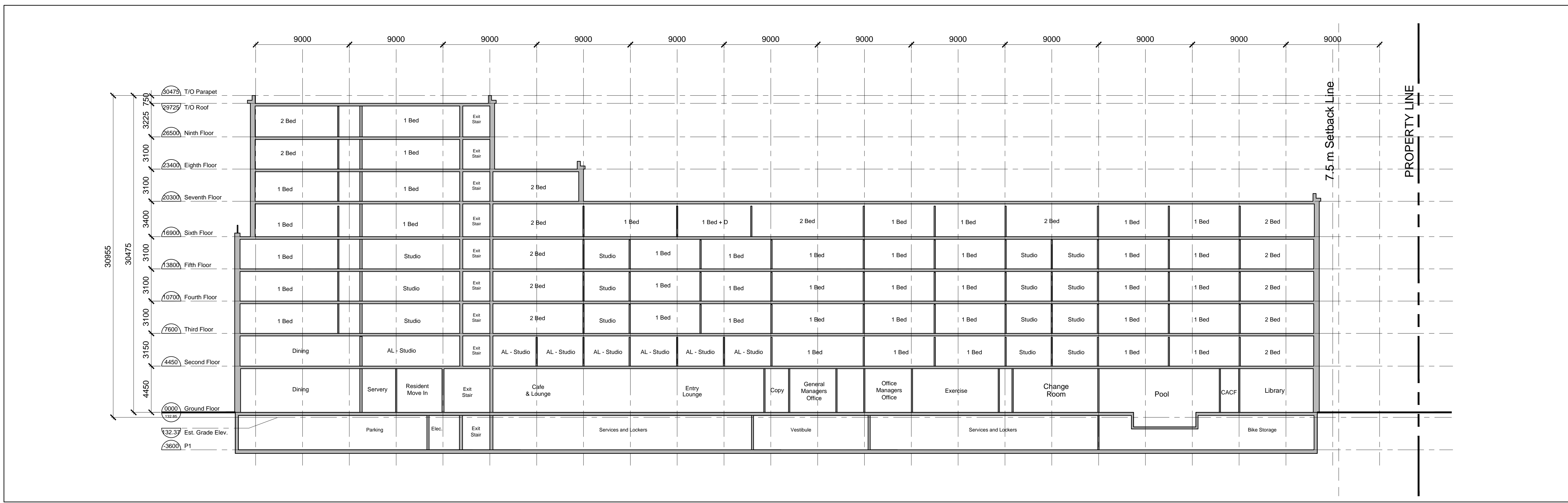
1 Section A-A A302 Scale: 1:200
