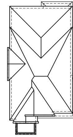
ROOF PLAN ELEV. 'B' N.T.S.
