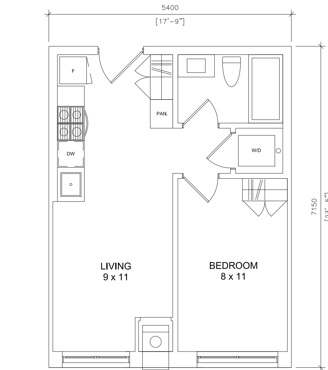
1 1br STANDARD UNIT (415 sf) A-5.1 SCALE: 1:50
