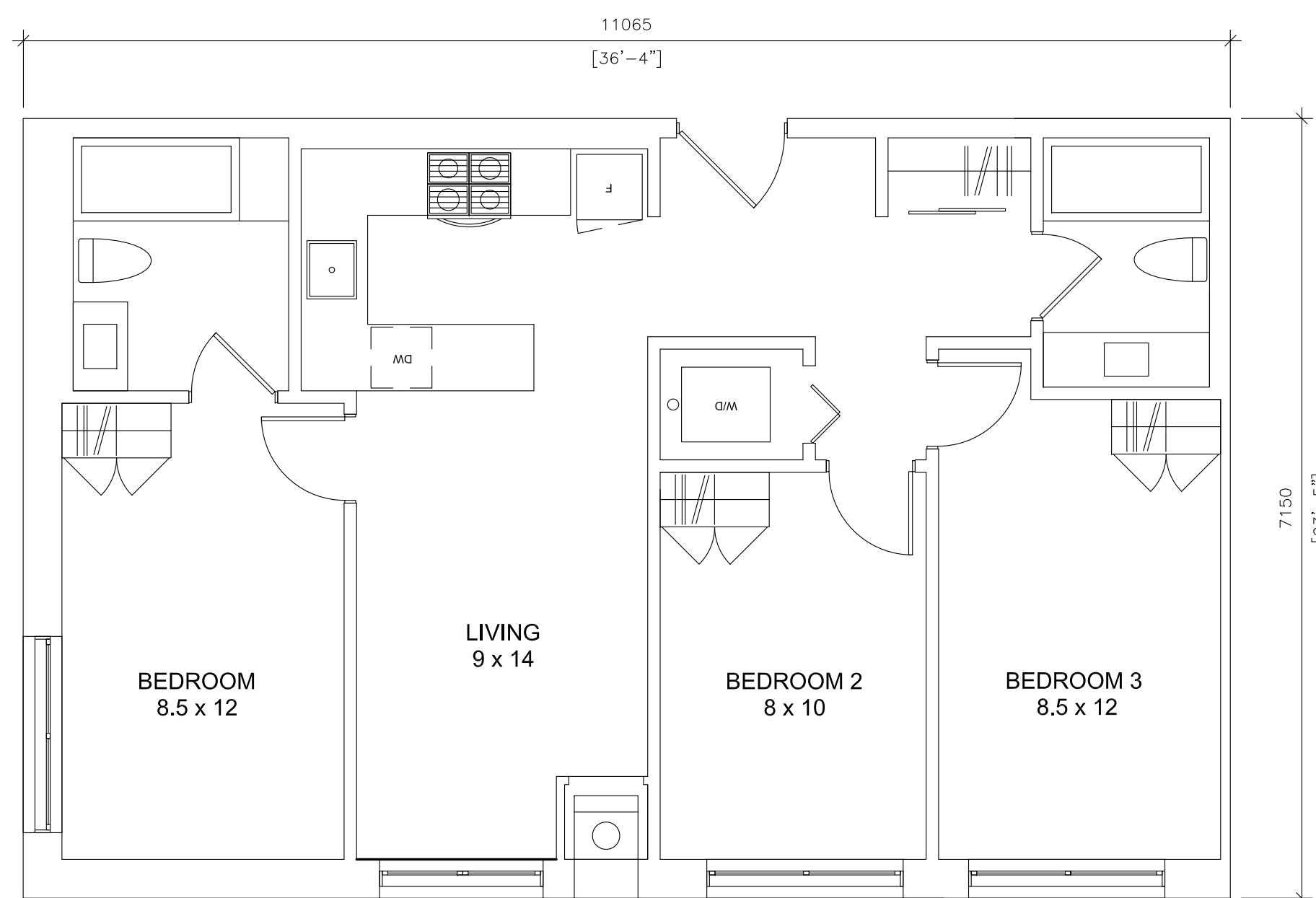
3 3br STANDARD UNIT (850 sf) A-5.1 SCALE: 1:50
