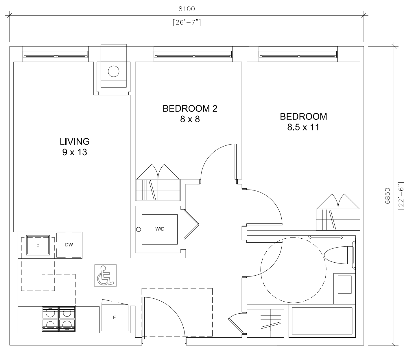
5 2br ACCESSIBLE UNIT (600 sf) A-5.1 SCALE: 1:50
