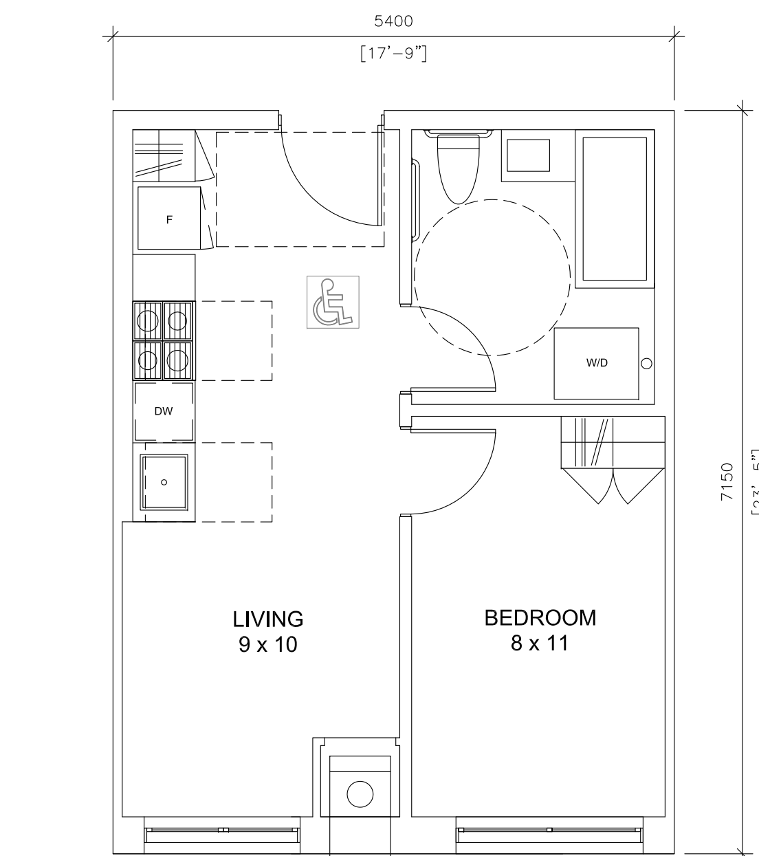
4 1br ACCESSIBLE UNIT (415 sf) A-5.1 SCALE: 1:50
