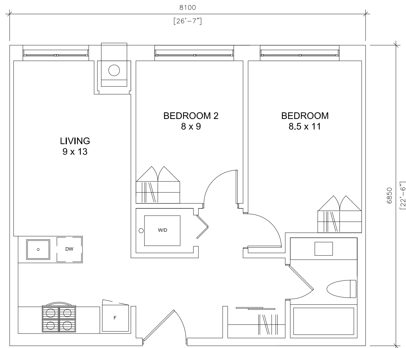
2 2br STANDARD UNIT (600 sf) A-5.1 SCALE: 1:50
