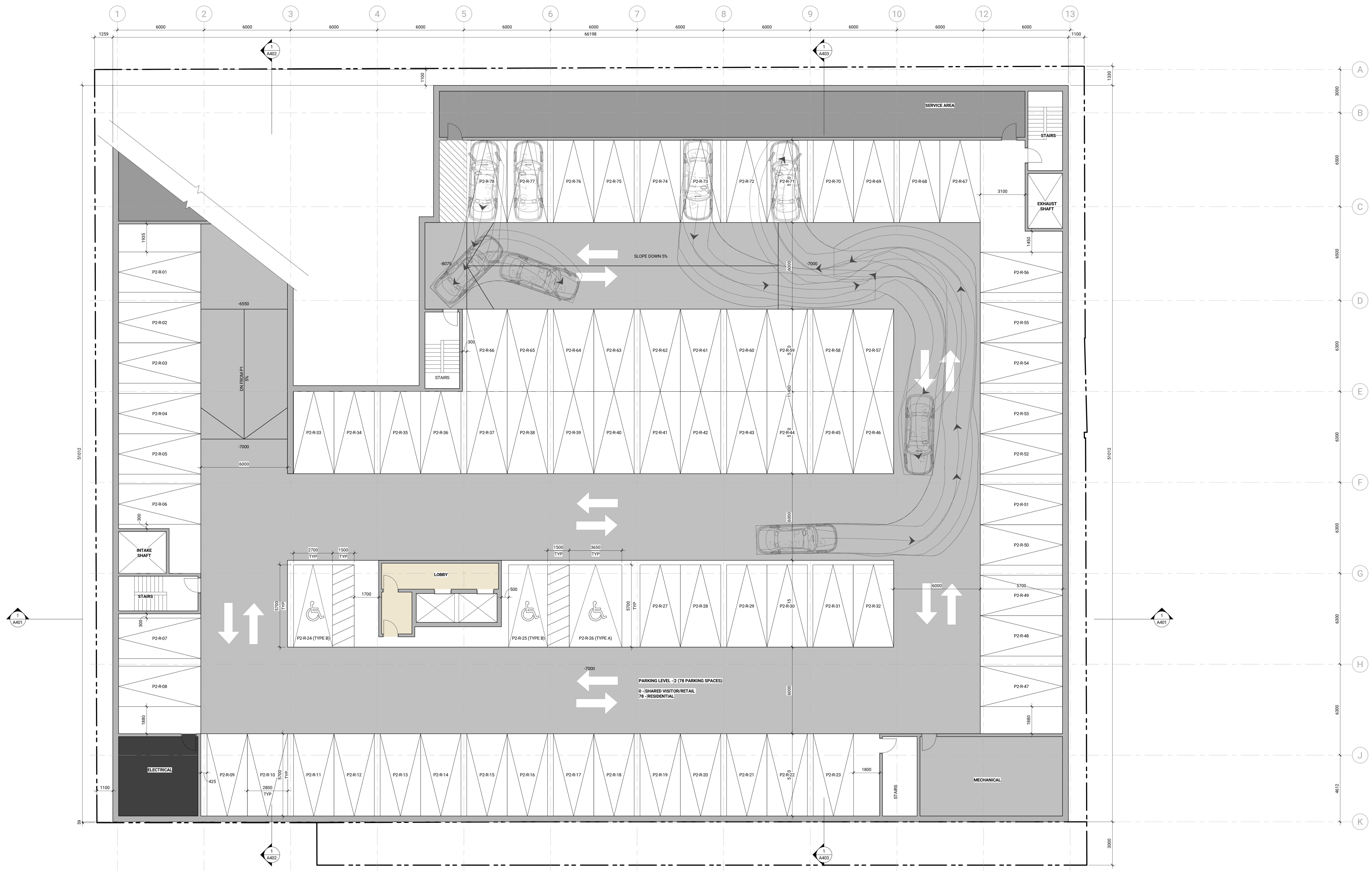
A-Level P2 1:100 1 A099
